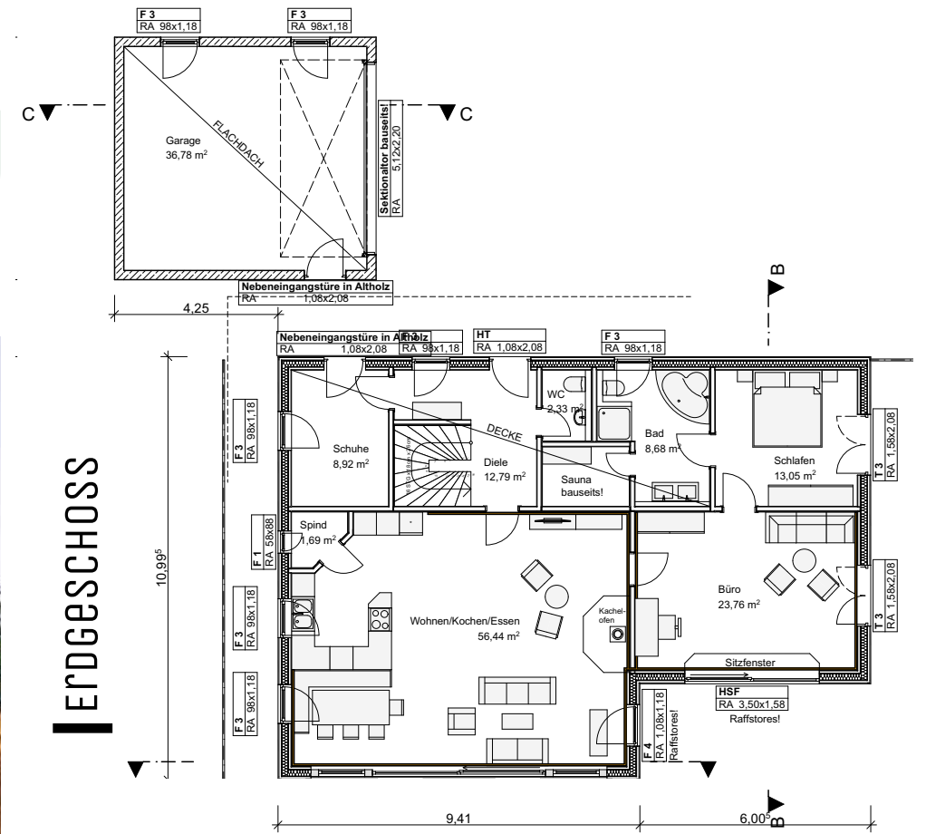
Die Grundrisse sind beispielhaft und können nach Ihren Wünschen geändert werden.
